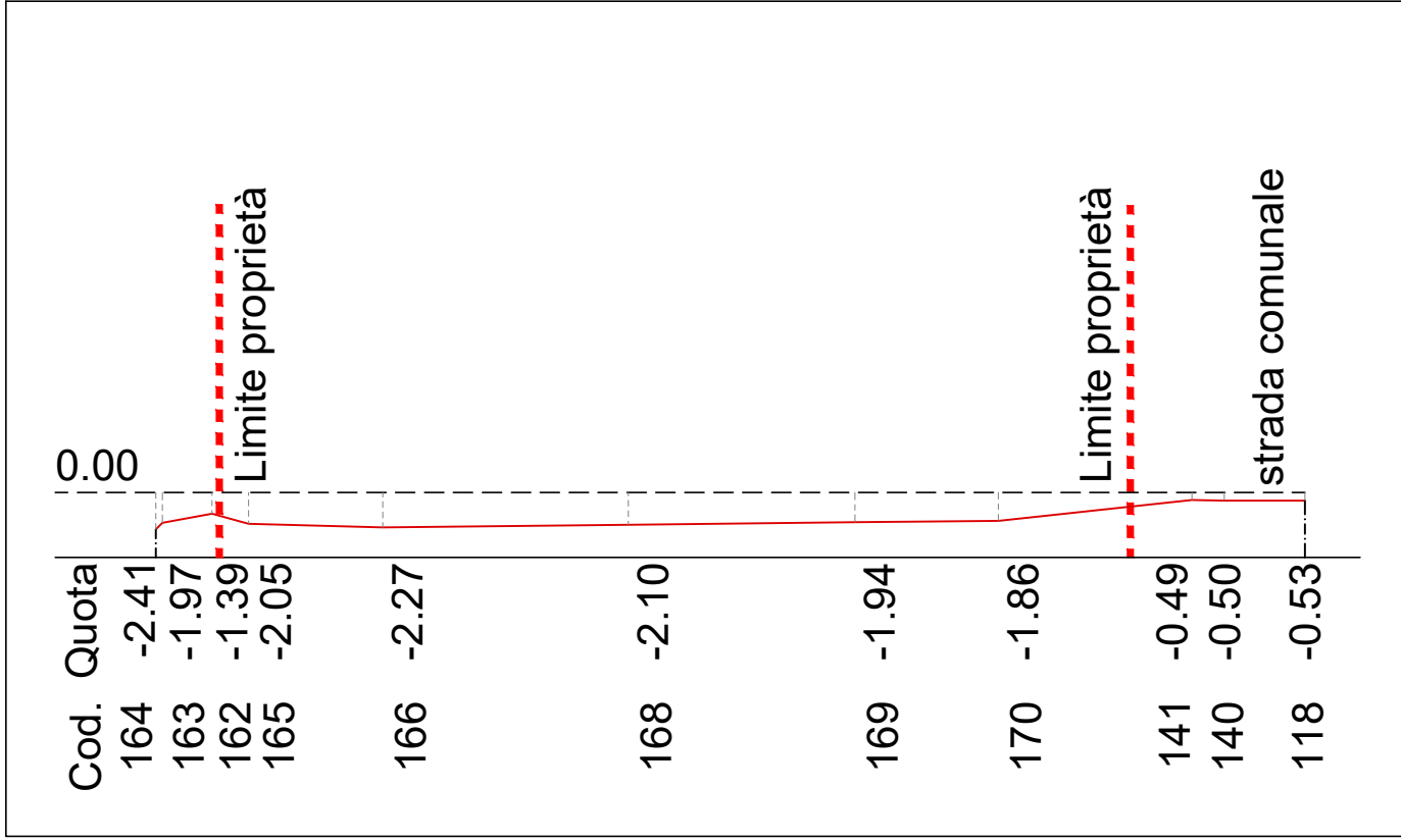
SEZ. A-A' 1:500
